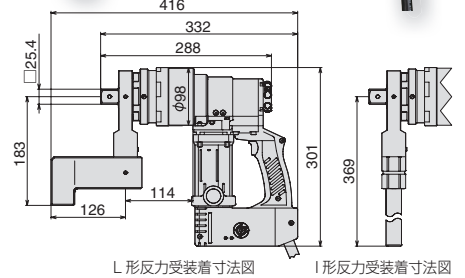
GST211T (Q 形 & I 形反力受装着)
