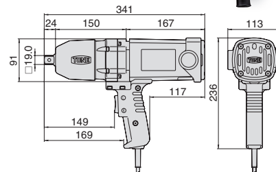
寸法図 (ソケット非装着)
