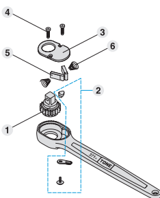
371 部品展開図
