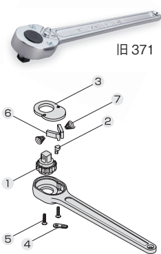
旧 371 部品展開図
