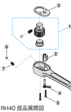
RH40 部品展開図
