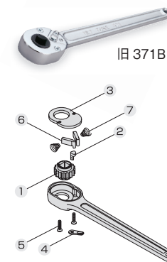
旧 371B 部品展開図
