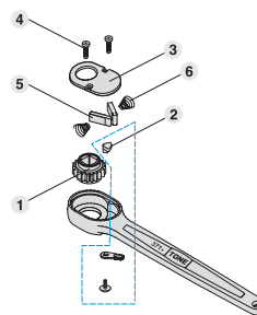
371B 部品展開図
