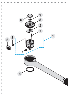
RH31 部品展開図
