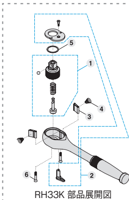
RH33K 部品展開図
