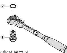
RH3VHW 部品展開図
