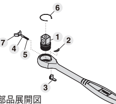
RH3CH 部品展開図
