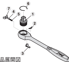
RH3H 部品展開図
